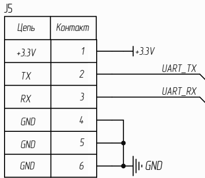
UART
