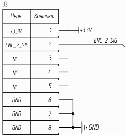
Датчик положения механизма фиксации
